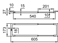
Телескопічний тримач
