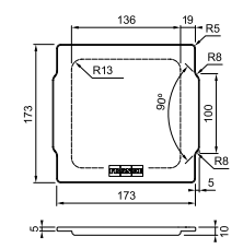
Бамбукова кришка
