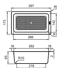
Великий коландер
