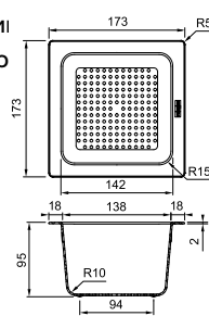
Великий коландер
